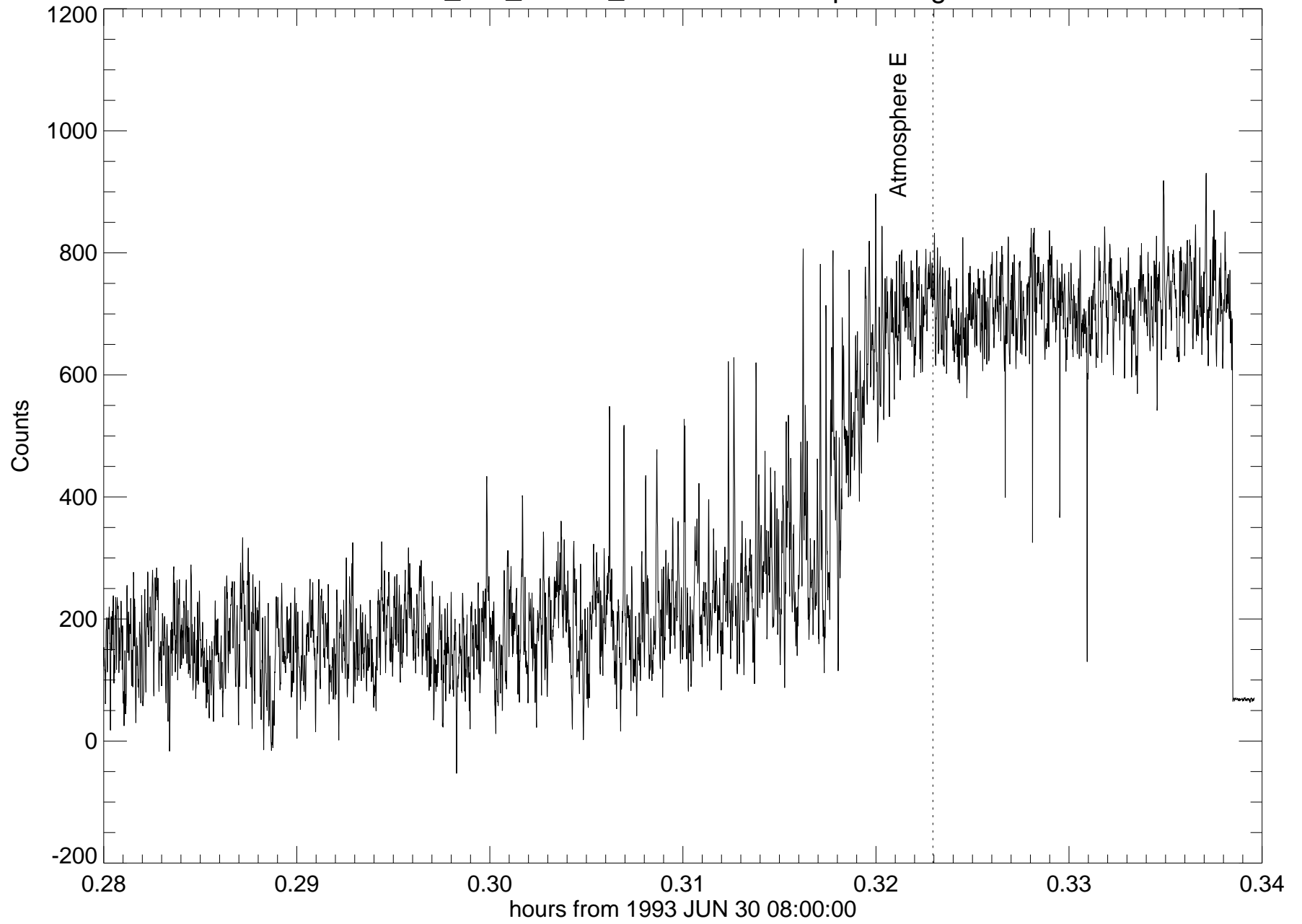
u9539_ctio_400cm_2200nm - atmosphere egress
