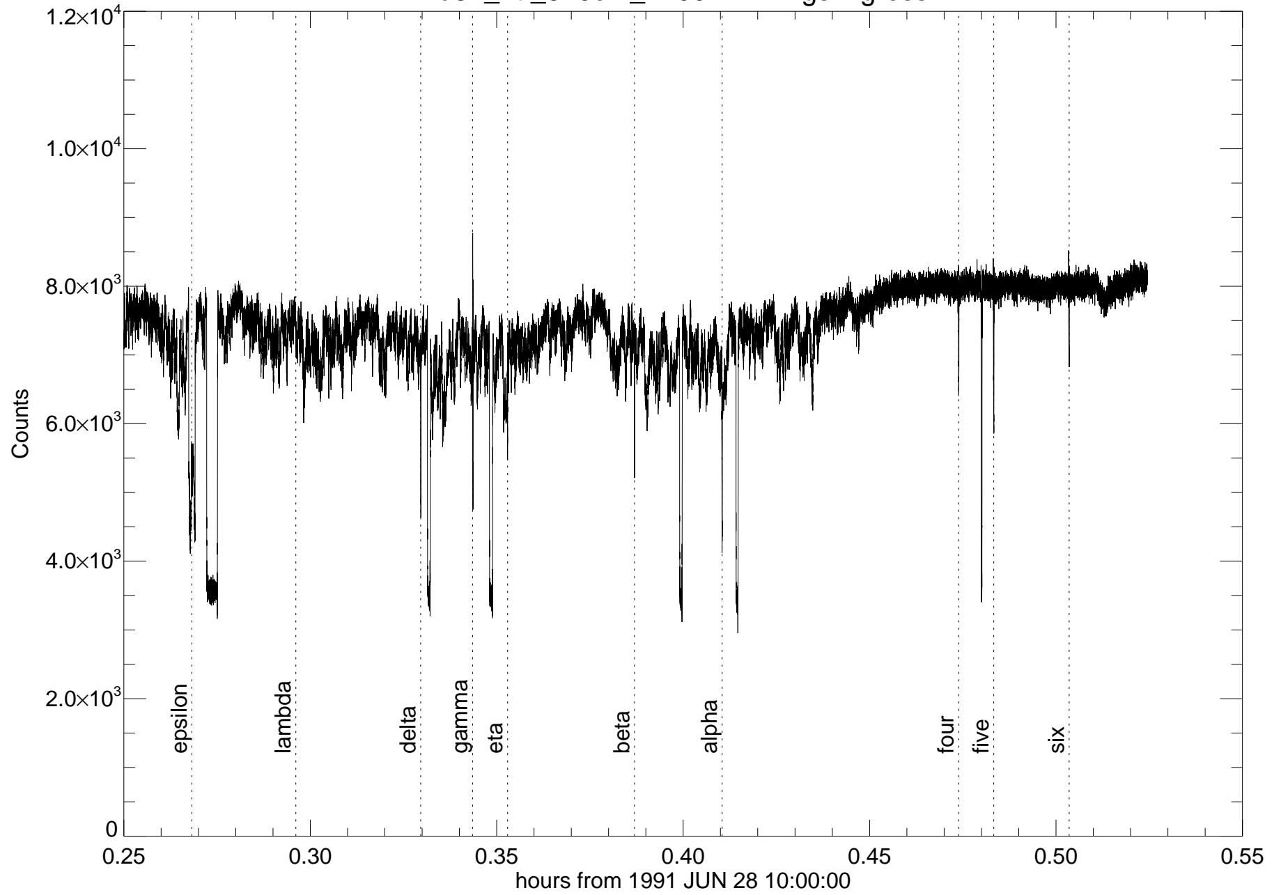
u84_irtf_320cm_2200nm - rings ingress
