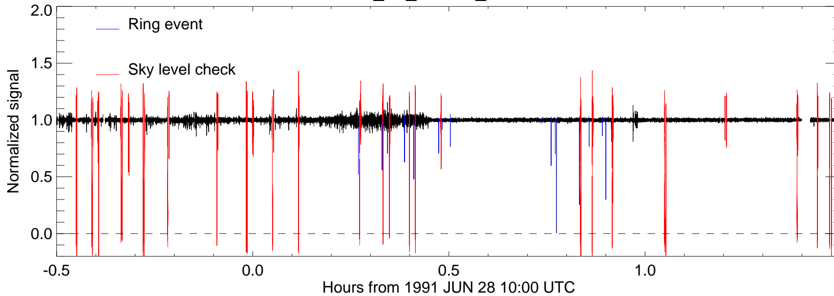
u84_irtf_320cm_2200nm
