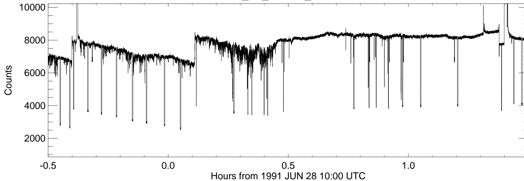
u84_irtf_320cm_2200nm
