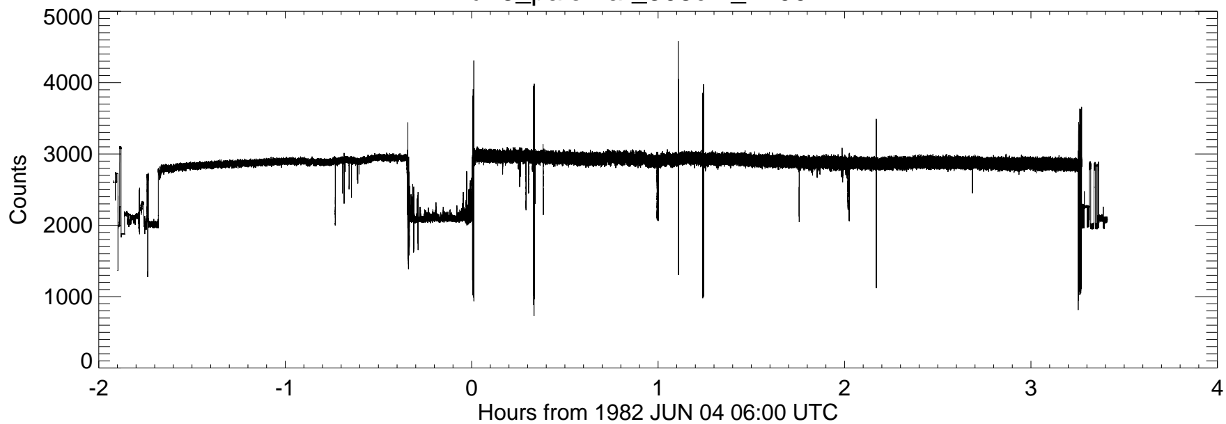
u16_palomar_508cm_2200nm
