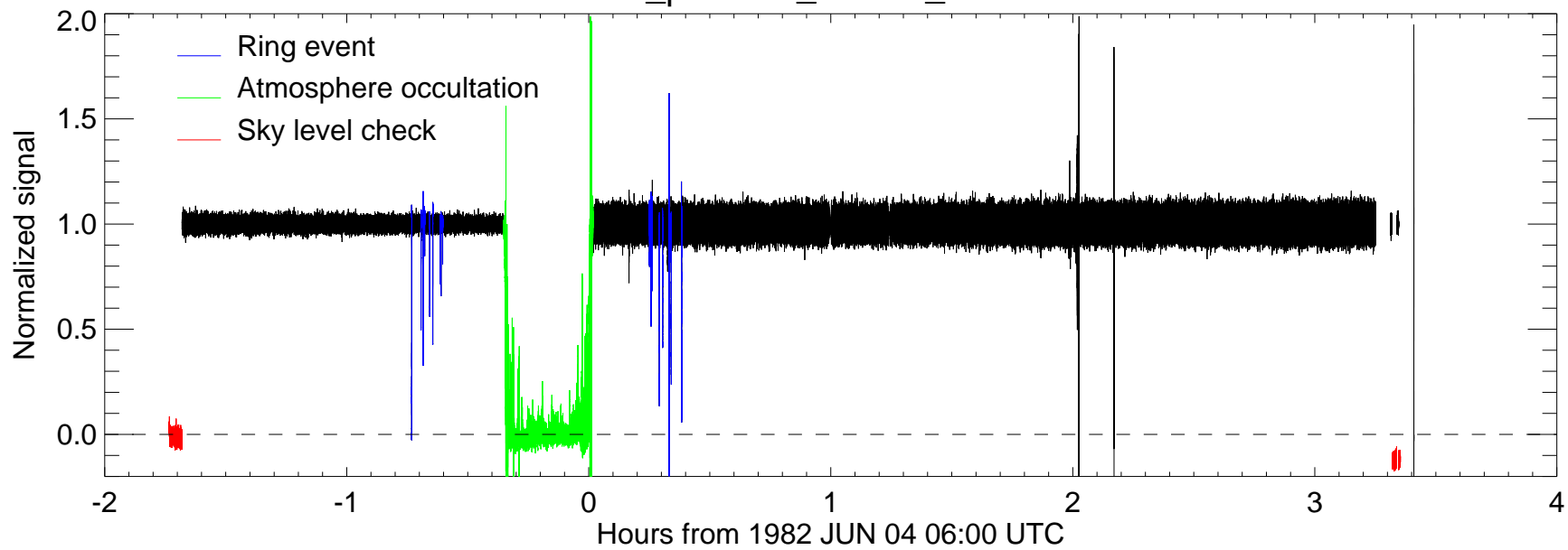
u16_palomar_508cm_2200nm
