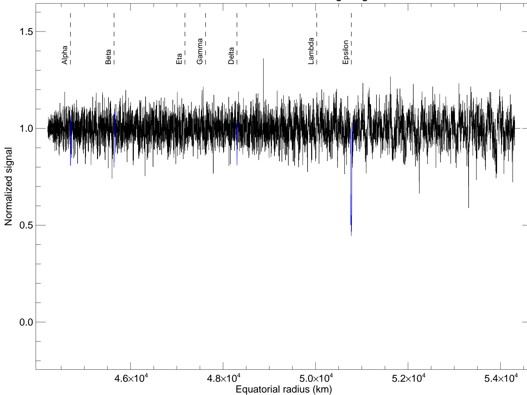
u11_ctio_400cm_2200nm rings ingress
