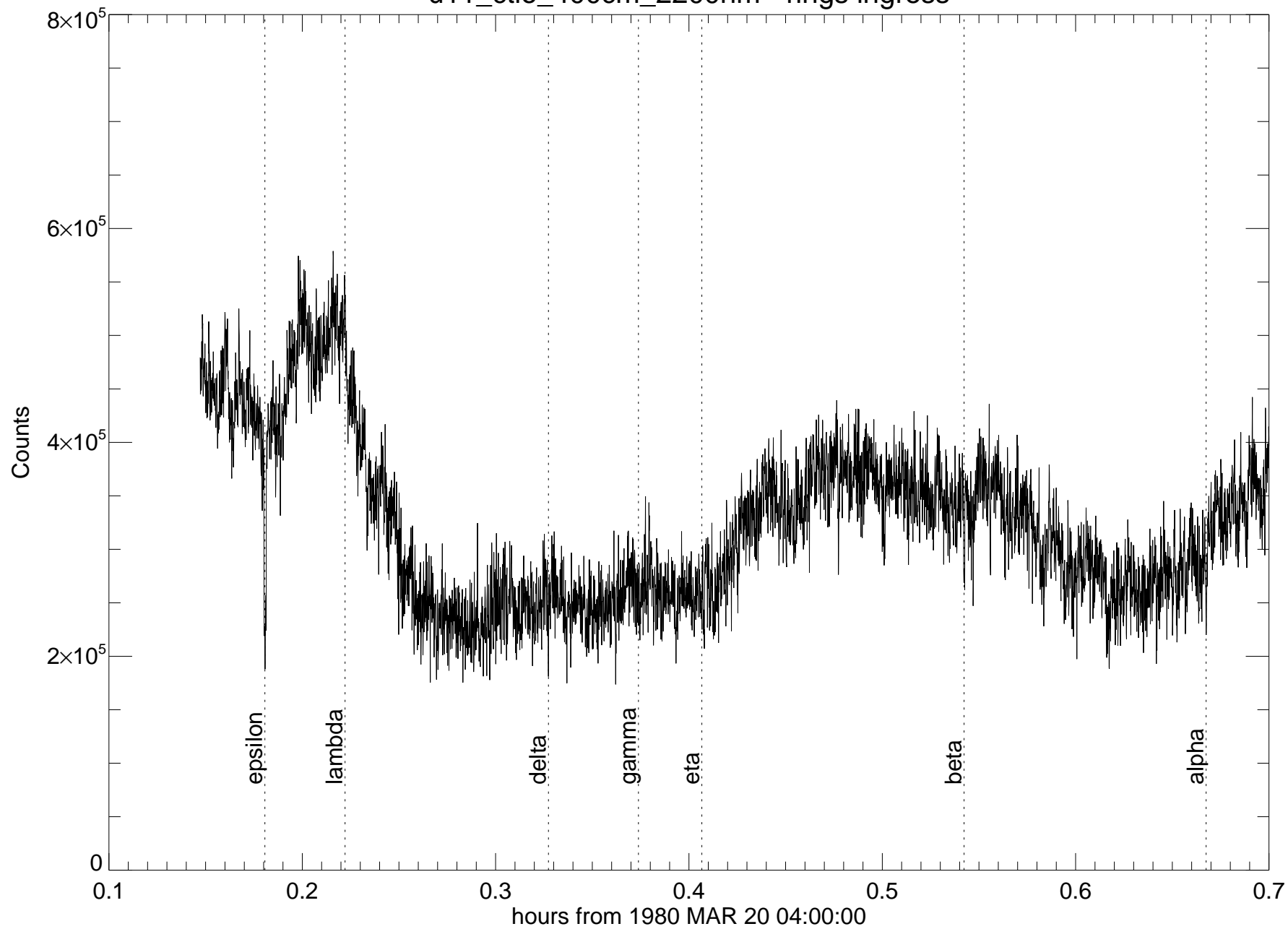
u11_ctio_400cm_2200nm - rings ingress
